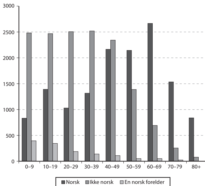
Figur 1 Befolkningsdiagram 2012
